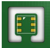
图10 AHT20 印刷电路板俯视图，图中加入铣削狭缝的设计，可以将热传递降到最小。
