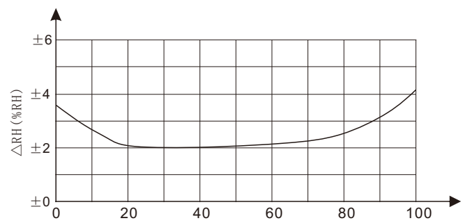
湿度误差图
