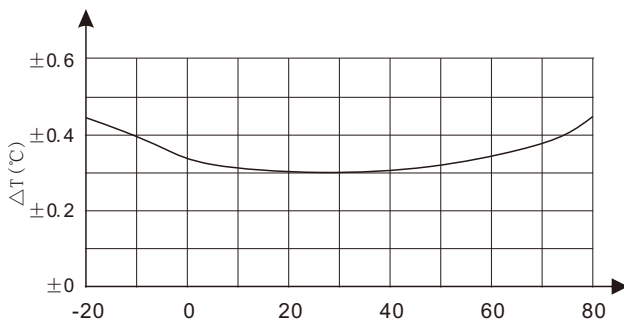
温度误差图
