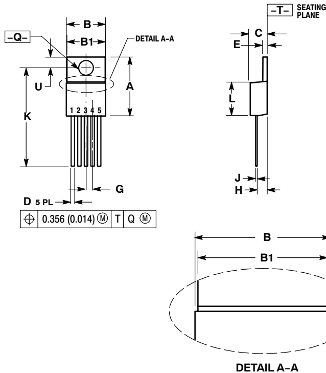
DETAIL A-A
