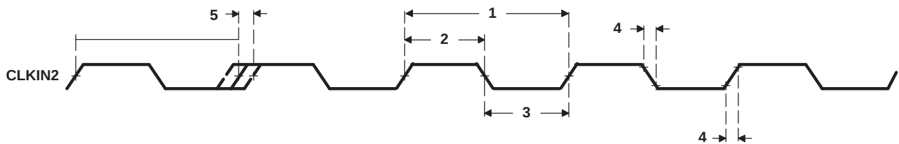
Figure 7-30. CLKIN2 Timing
